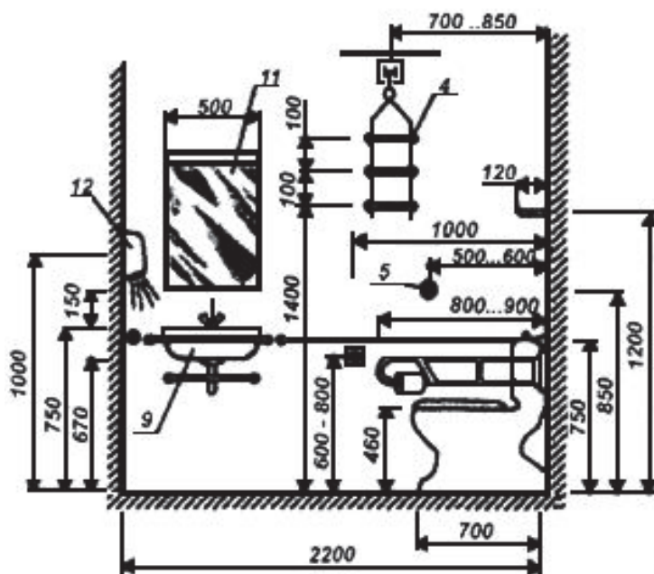
Разрез А-А
